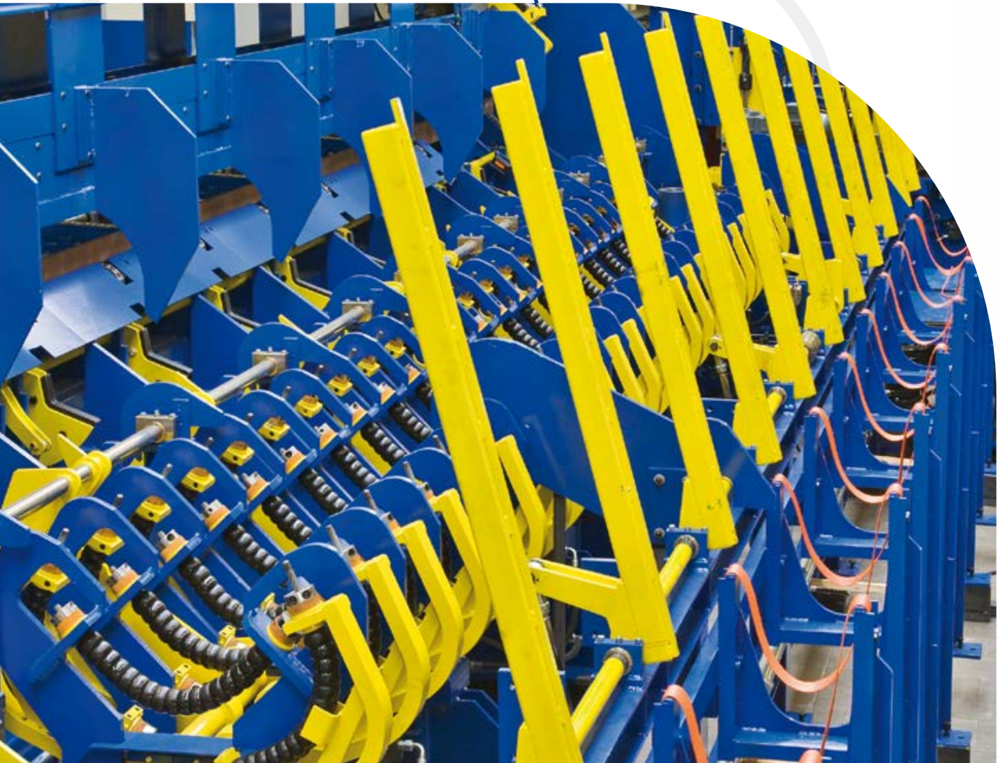
Vereinzelung / Einlaufbahn für Stahlstangen Separation system / entry roller path for steel bars
