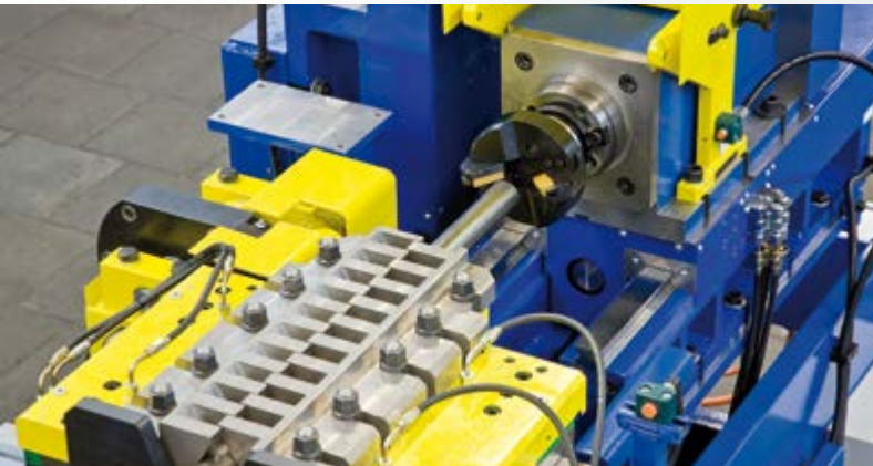
Fasanlage für Stahlstangen Chamfering machine for steel bars
