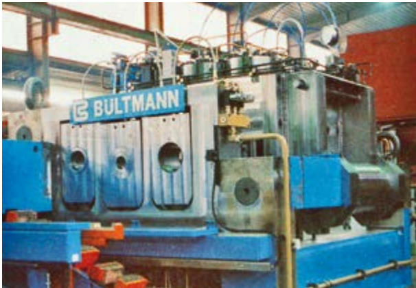
3-fach-Einschubvorrichtung für Rund-, Sechskant- und Vierkantstangen aus Edelstahl Triple push-in device for rounds, hexagons and squares made from special steel
