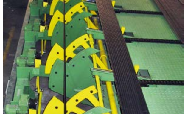
Quertransport zwischen einer Schälmaschine und einer 2-Walzen-Richtmaschine
