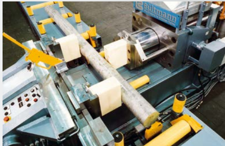
3000 kN Richtpresse für Aluminiumstangen und -profile 3000 kN straightening press for aluminium bars and profiles
