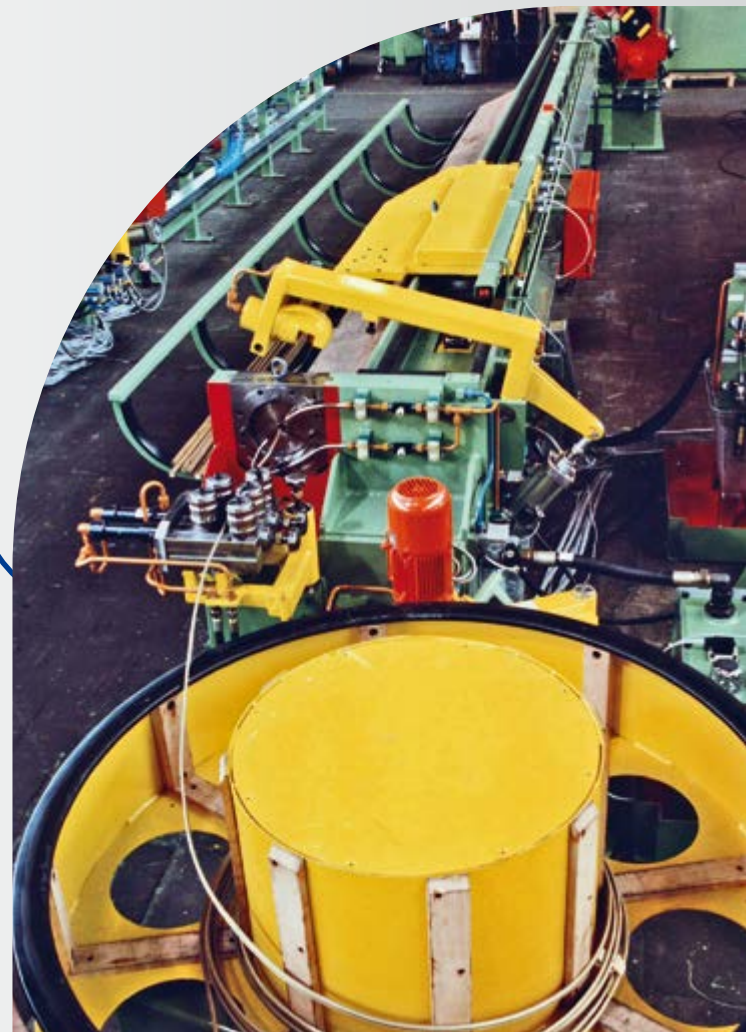
1-fach-Stangenziehanlage für Messingstangen mit Abcoiler, Vorrichtmaschine und Abschervorrichtung Single drawing line for brass bars with uncoiler, pre-straightener and shear-off device
