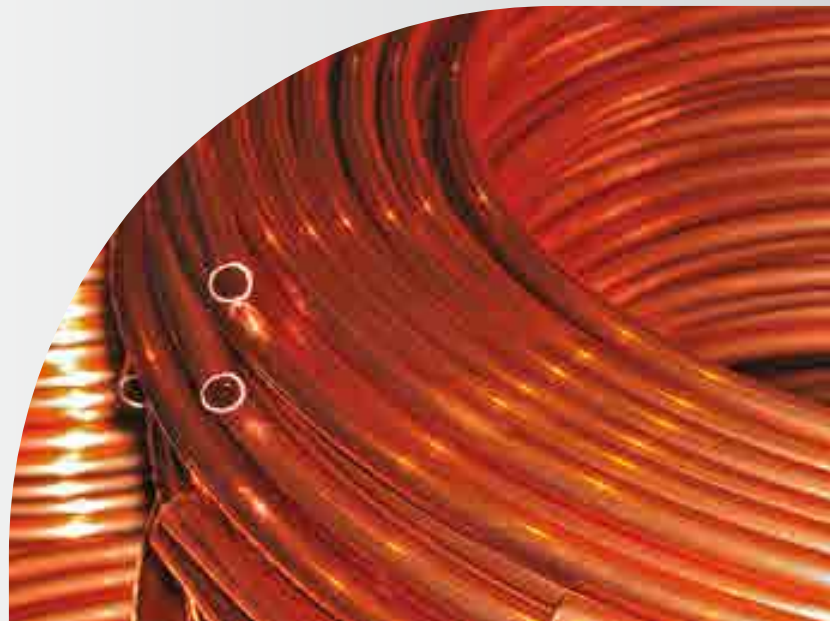
Aufcoiler im Pressenauslauf für kupferlegierte Rohre und Profile Coiler for copper-alloyed tubes and profiles, arranged in the runout of an extrusion press
