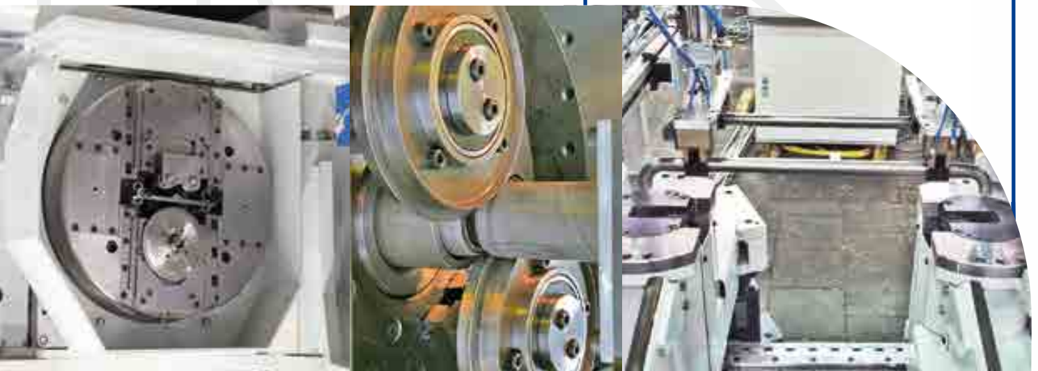
1-fach-Spanlostrennanlage für hochwertige Edelmetallrohre Single chipless cutting unit for high-grade precious metal tubes
